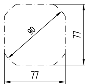
Maße für Montagewand
