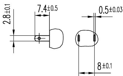
Maße für Steckeranschluß
